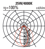
ONEline 1.2 INTENS Systemleuchte
