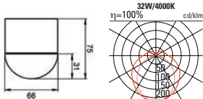
ONEline 1.5 RUND Systemleuchte
