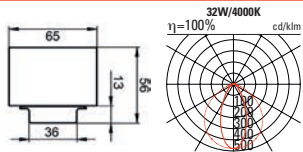
ONeline 1.5 INTENS Systemleuchte
