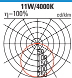
GIULIA 200 Anbauleuchte mit LED-Modul
