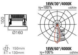
TAKEO T150 ohne Betriebsgerät (500mA)
