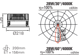
TAKEO T200 ohne Betriebsgerät (700mA)
