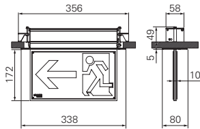
Deckenöffnung 324x60x49mm Abdeckplatte 338x80x5mm
