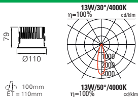
TAKEO T100 ohne Betriebsgerät (350mA)
